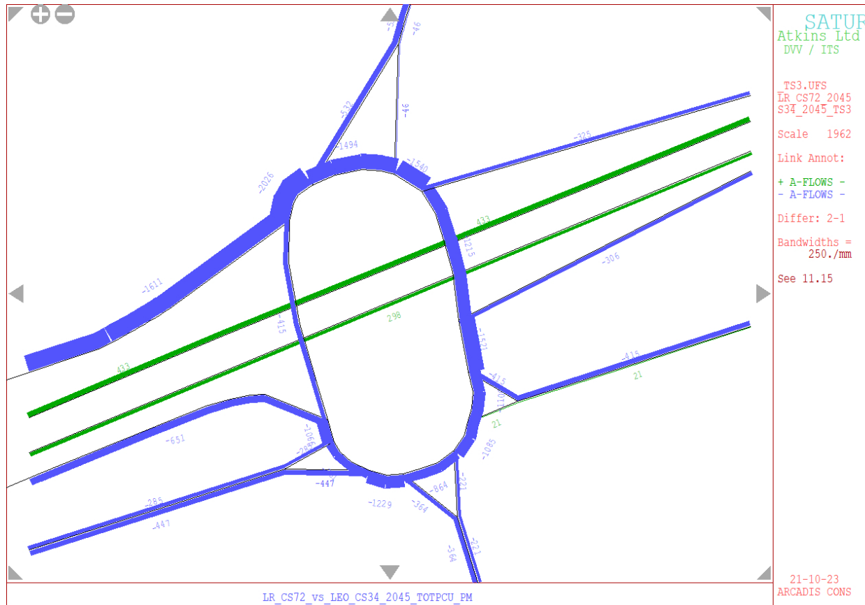
Plate N.13 2045 PM plots VISSIM delays hard coded into SATURN, Orsett Cock
