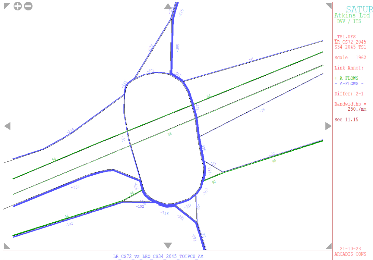
Plate N.10 2045 AM plots VISSIM delays hard coded into SATURN, Orsett Cock
